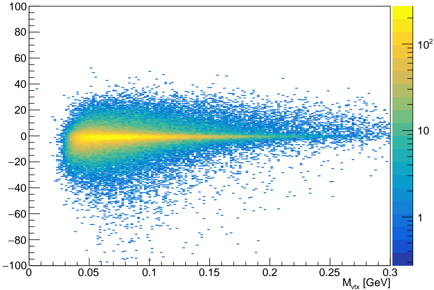
tridentL2L1-NoPosClust-EleClust_vtx_InvM_vtx_z_hh
