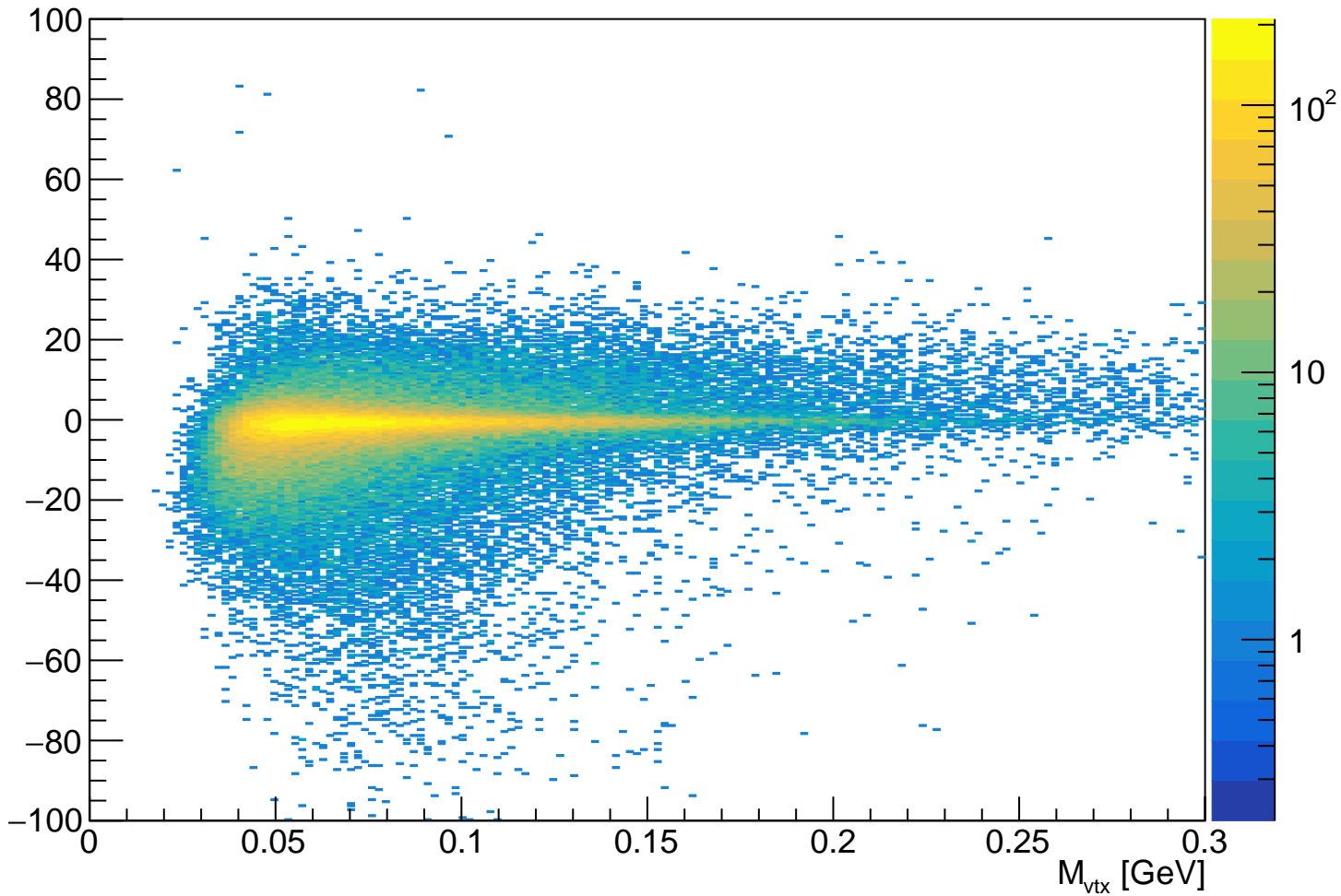
tridentL1L2-NoPosClust-EleClust_vtx_InvM_vtx_z_hh
