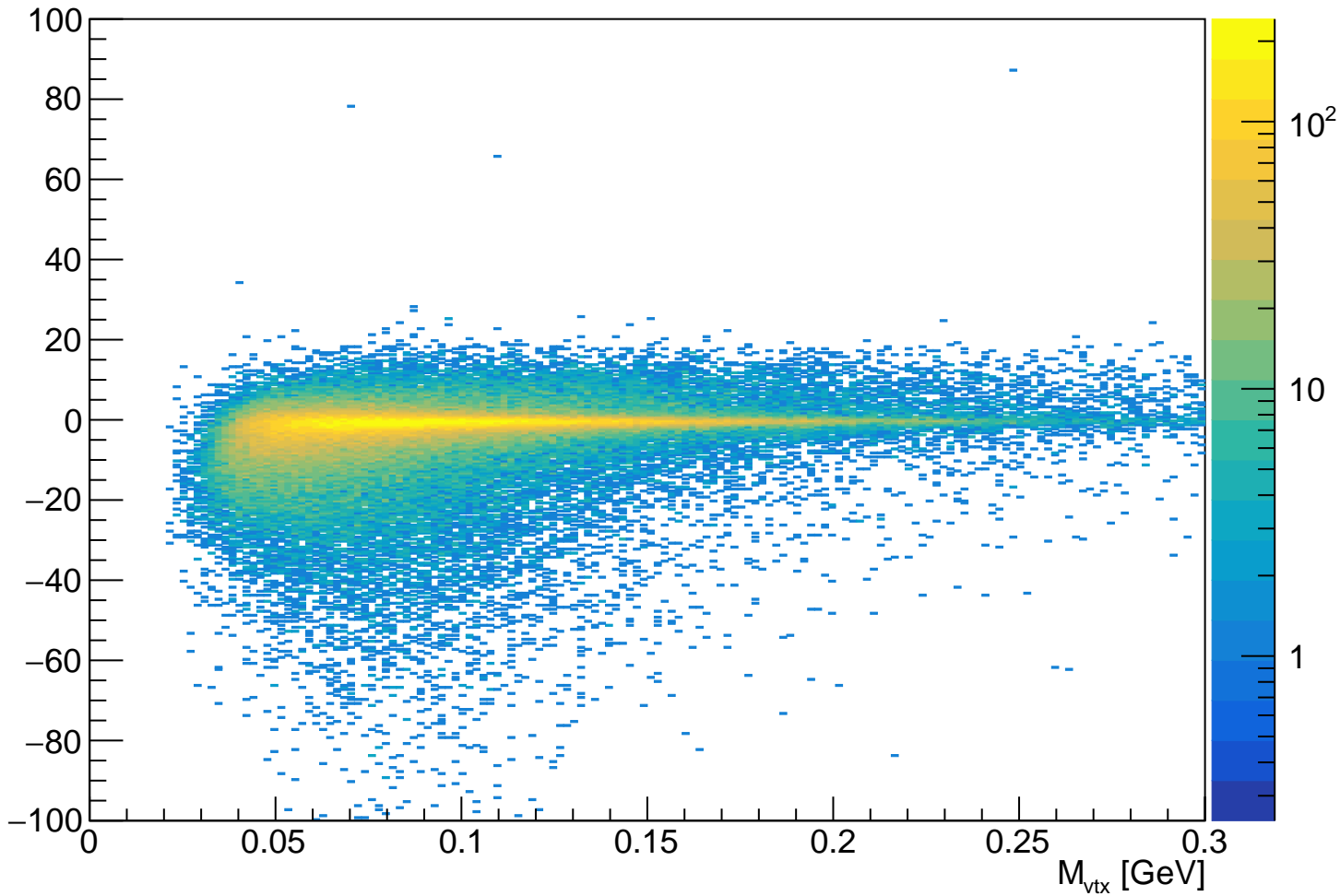
tridentL1L1-NoPosClust-EleClust_vtx_InvM_vtx_z_hh
