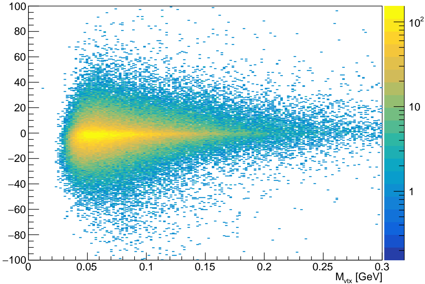
tridentNoInnerMatch-NoPosClust-EleClust_vtx_InvM_vtx_z_hh
