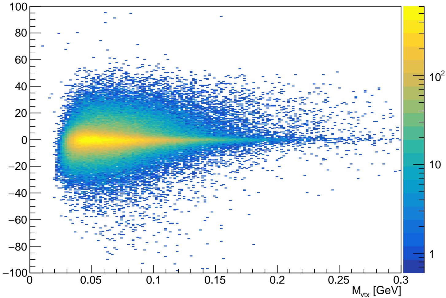
tridentL2L2-PosClust-NoEleClust_vtx_InvM_vtx_z_hh
