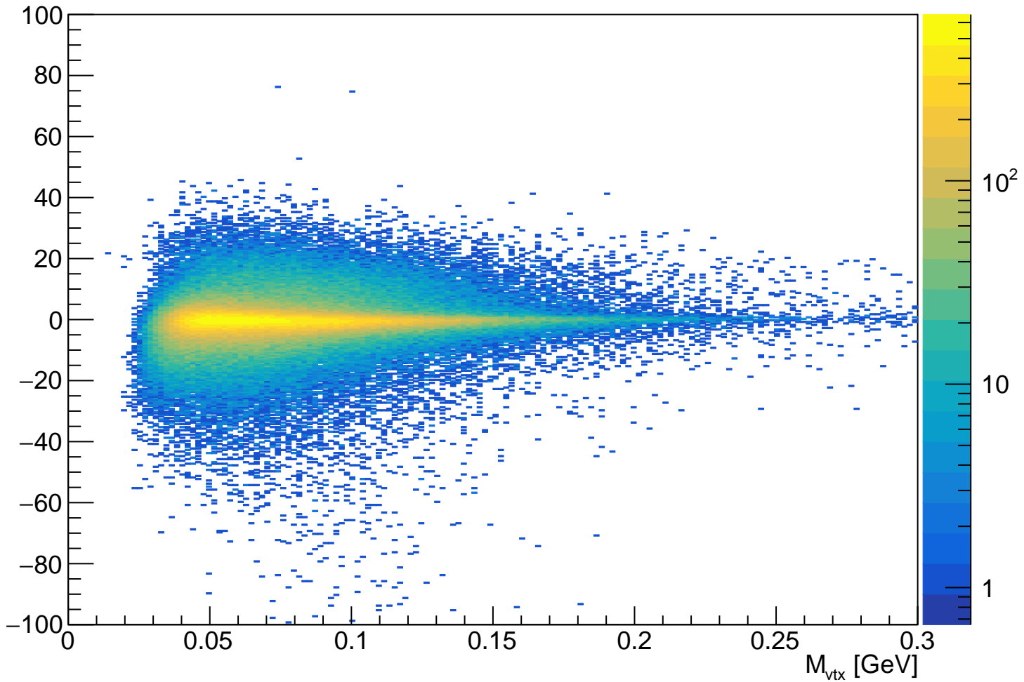
tridentL1L2-PosClust-NoEleClust_vtx_InvM_vtx_z_hh
