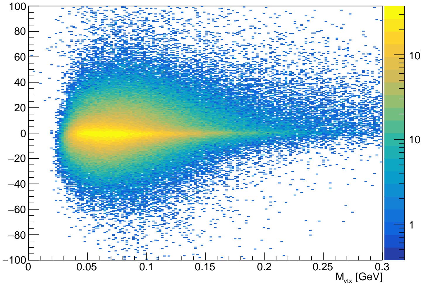
tridentNoInnerMatch-PosClust-NoEleClust_vtx_InvM_vtx_z_hh
