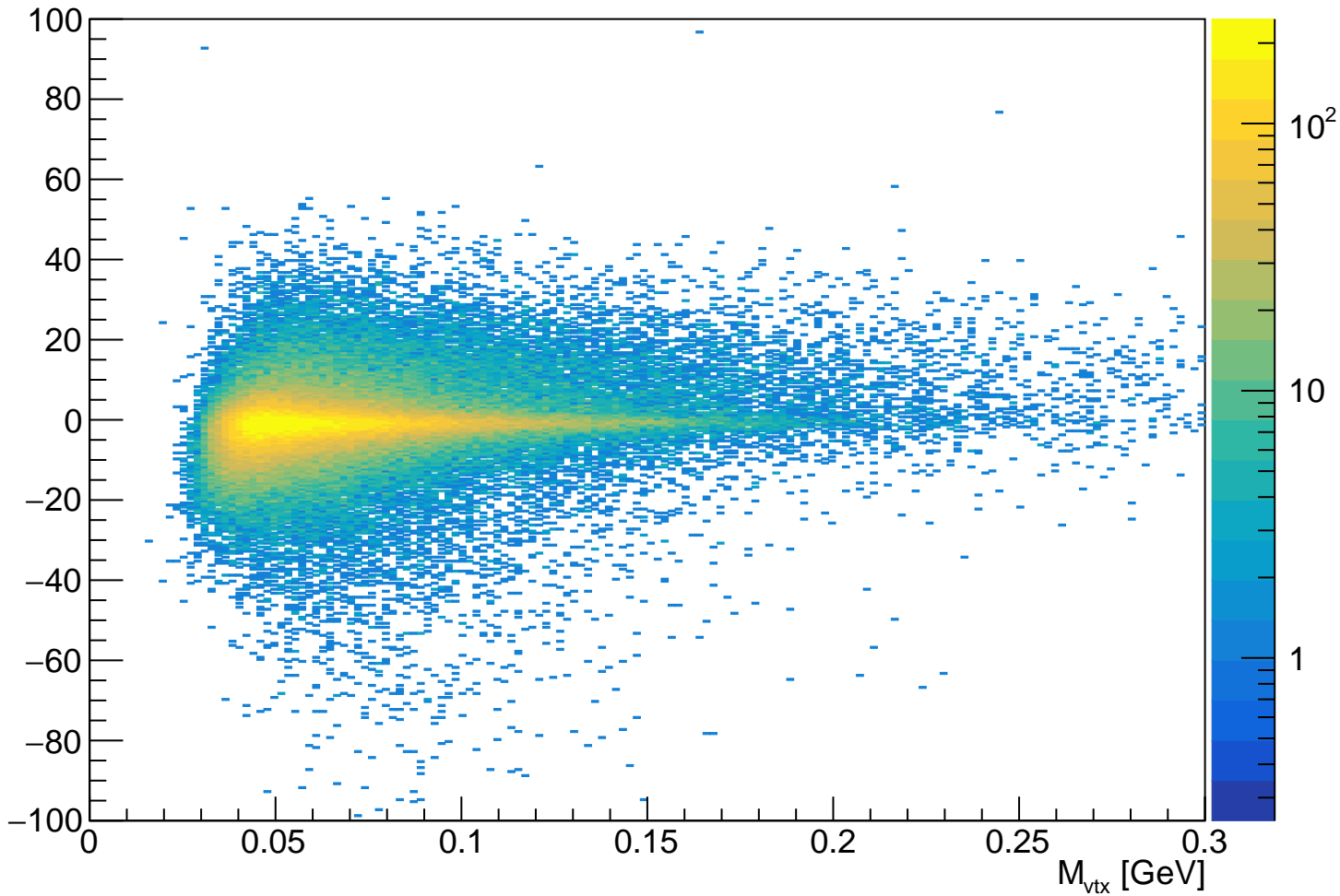
tridentL2L2-NoPosClust-EleClust_vtx_InvM_vtx_z_hh
