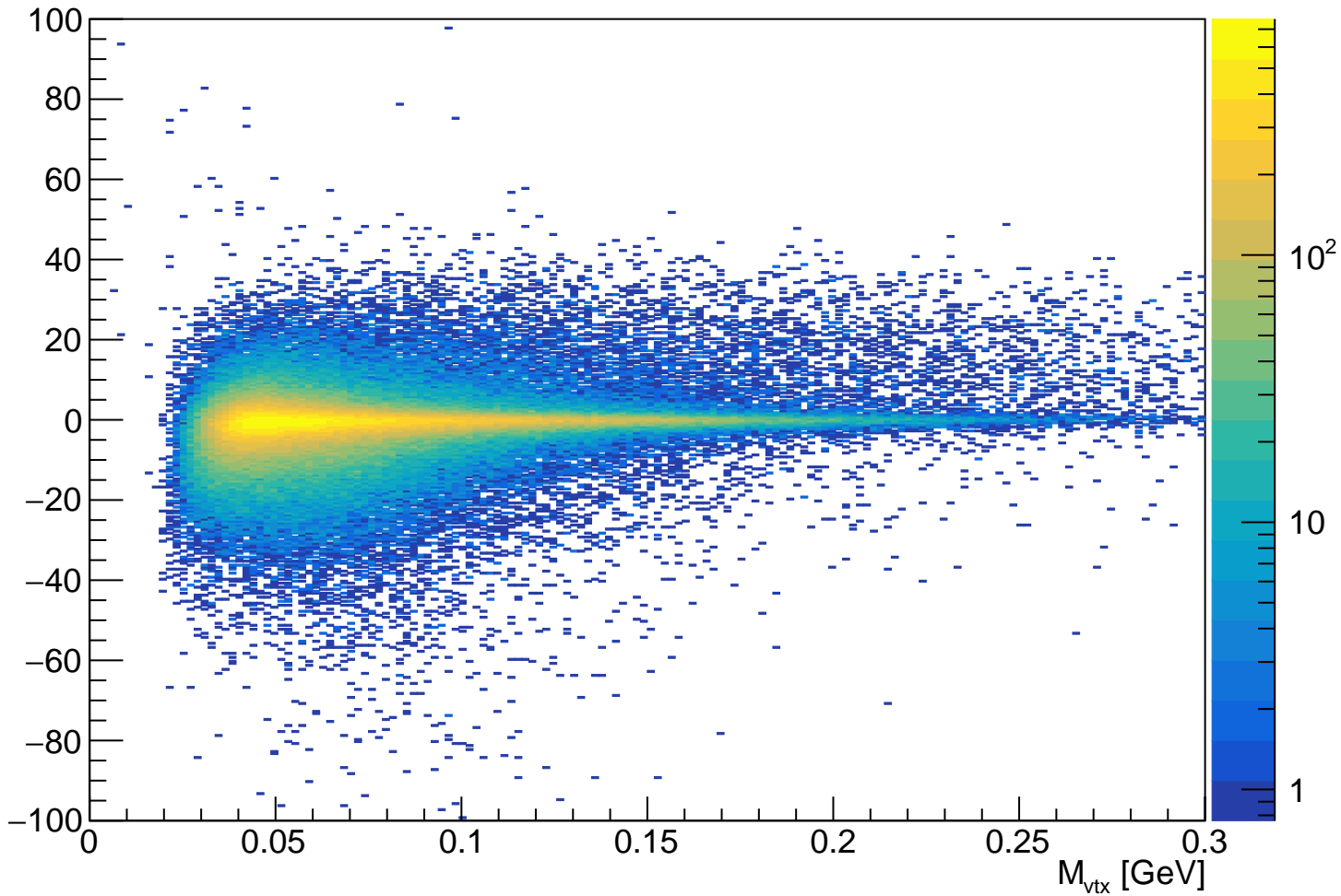
tridentL2L1-PosClust-NoEleClust_vtx_InvM_vtx_z_hh
