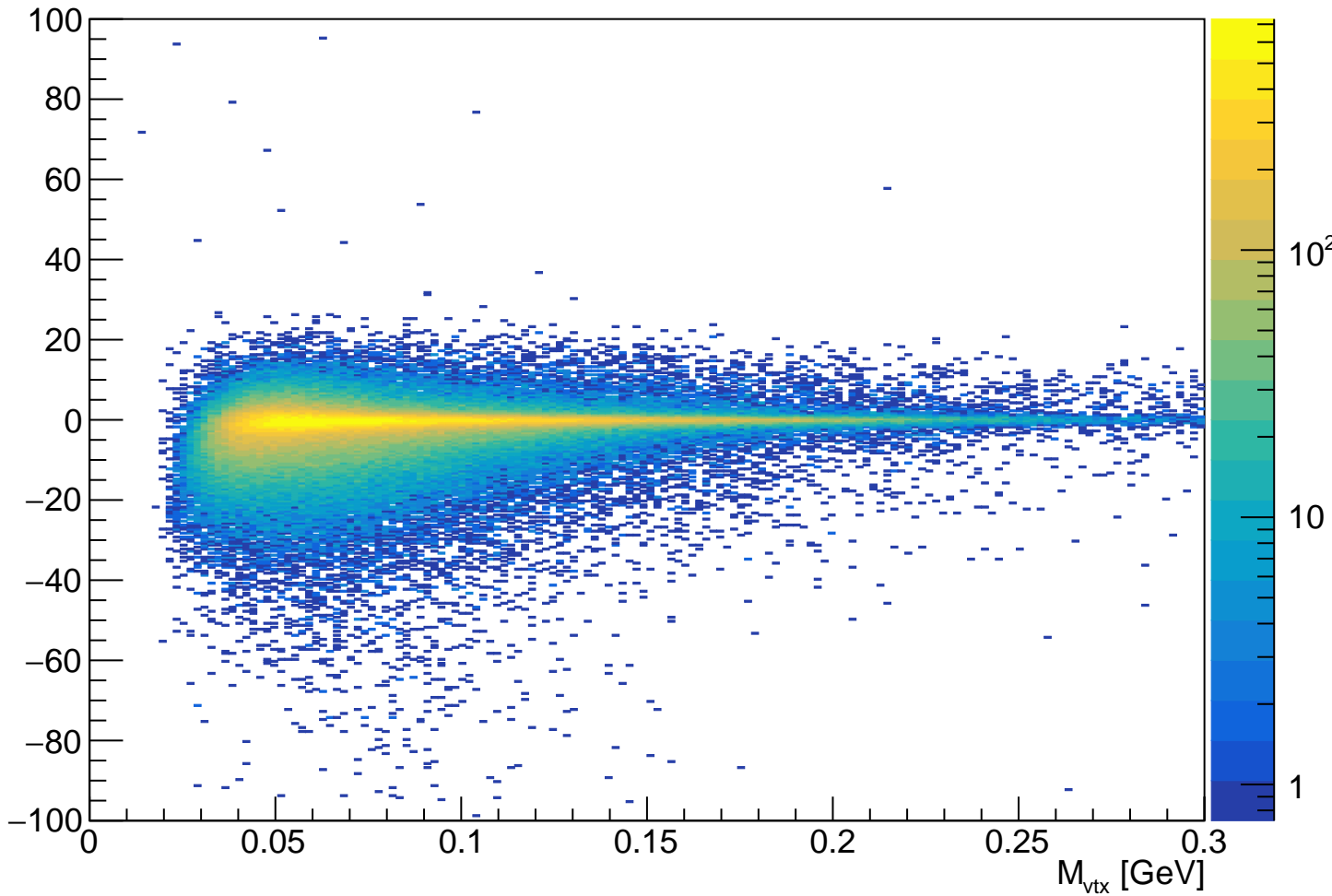
tridentL1L1-PosClust-NoEleClust_vtx_InvM_vtx_z_hh
