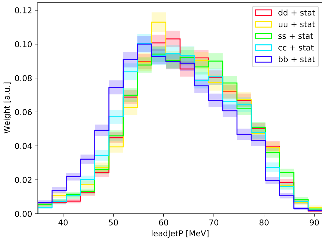
ILC-ILD : leadJetP (normalized)
