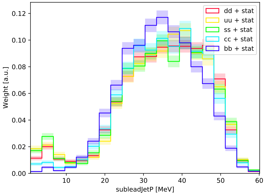
ILC-ILD : subleadJetP (normalized)
