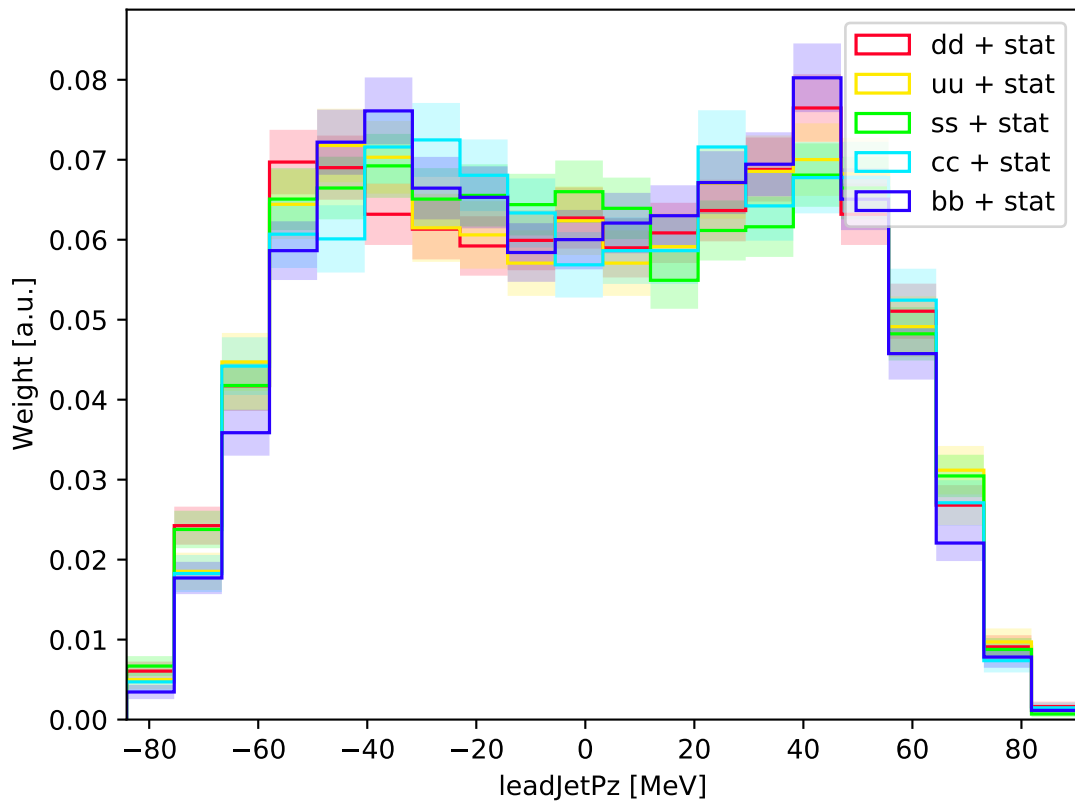
ILC-ILD : leadJetPz (normalized)
